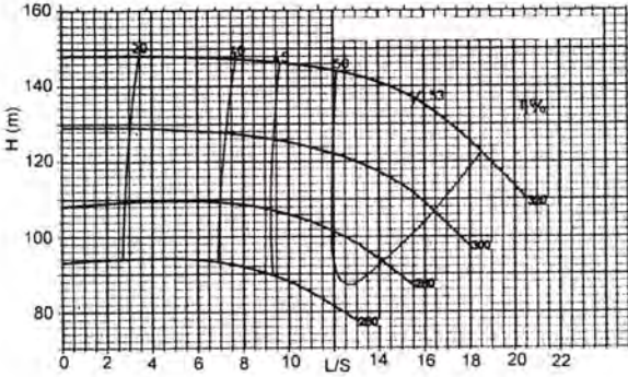
65-32 2 poles
