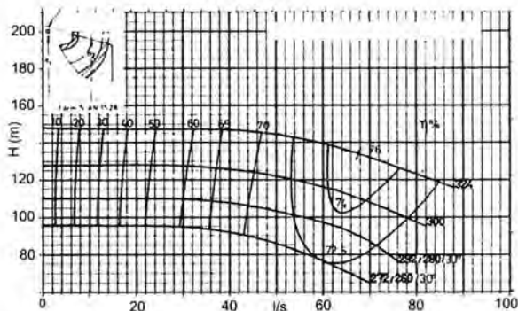
100-32 2 poles
