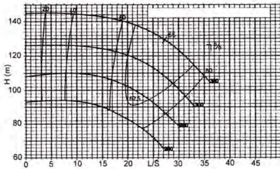
80-32 2poles
